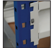
Fixation des longerons et goupille de renfort
