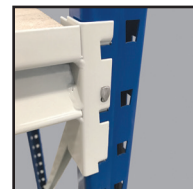
Fixation des longerons et goupille de renfort
