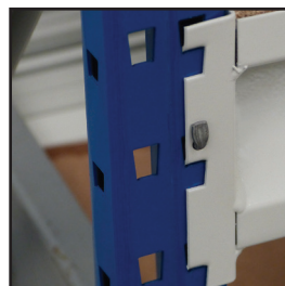
Fixation des longerons et des goupilles de sécurité
