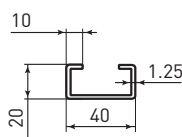
SECTION DU MONTANT
