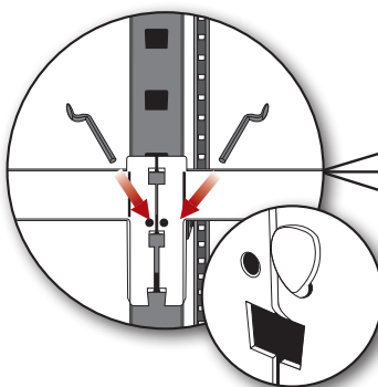
SYSTÈME DE GOUPILLES DE SÉCURITÉ POUR UN MEILLEUR RENFORT.
