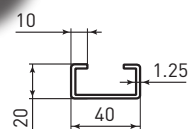
SECTIE VAN DE STEUNPILAAAR IN STAAL
