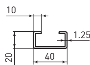
SECTIE VAN DE STEUNPILAAR IN STAAL
